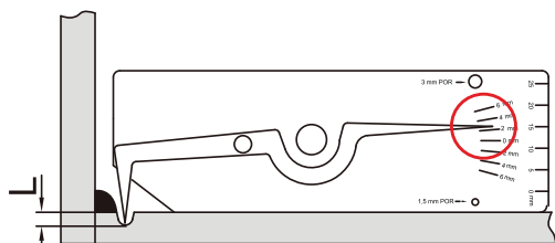
profundidad del socavado
