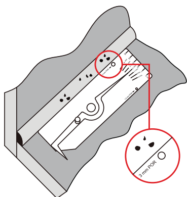
comparación del tamaño de la porosidad
