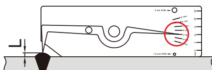
altura de la corona
