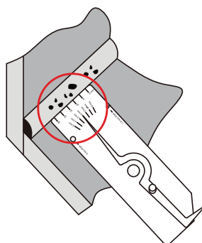
Cantidad de porosidad por 25 mm
